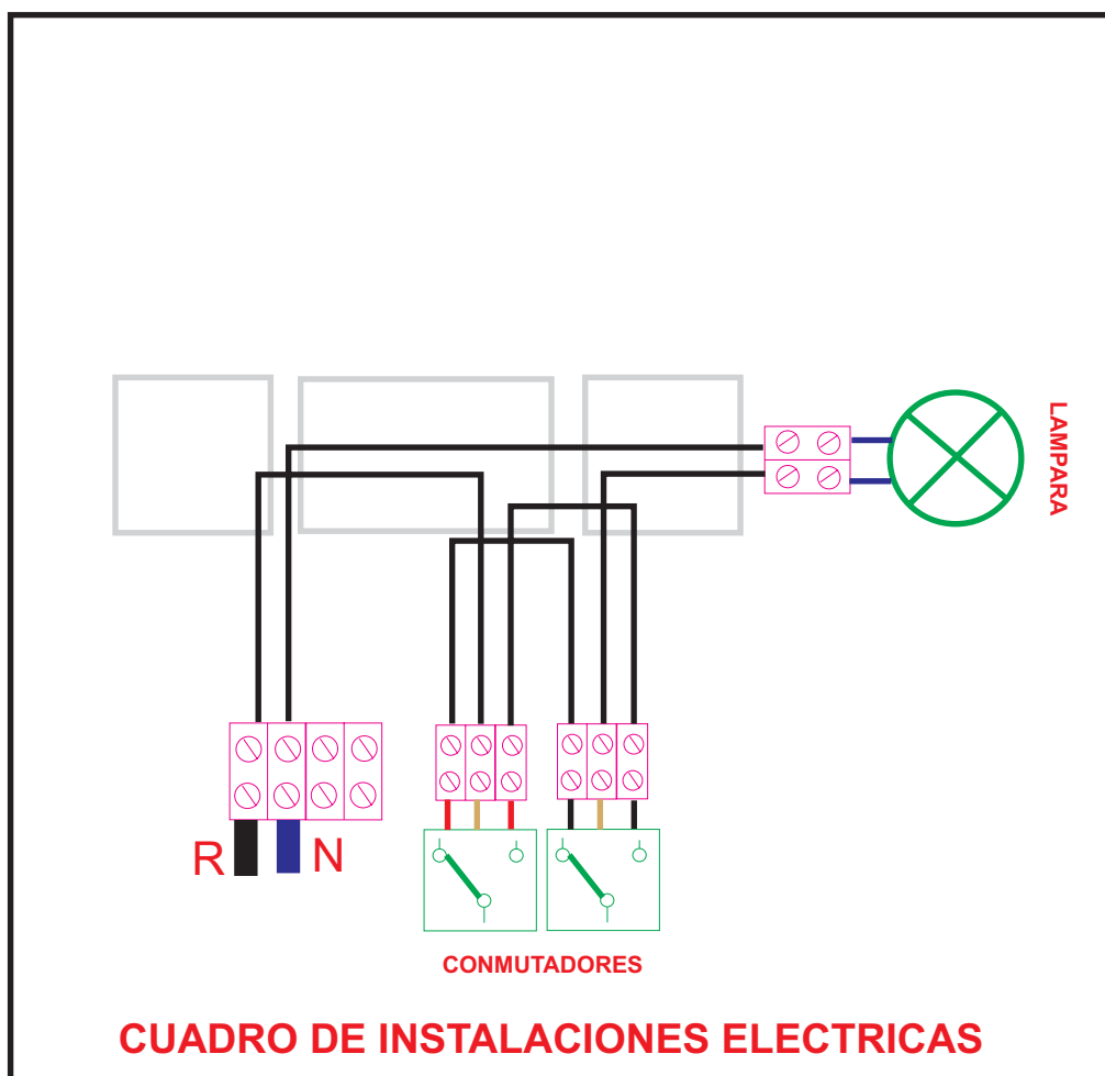
Esquema de conexiones
