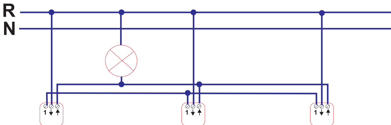
Esquema de funcionamiento
