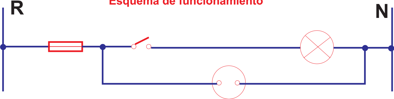
Esquema de funcionamiento
