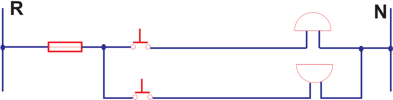
Esquema de funcionamiento
