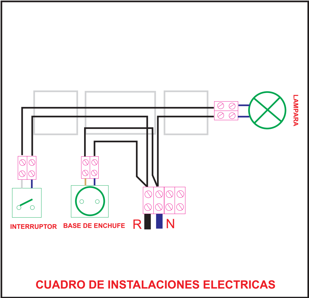
Esquema de conexiones
