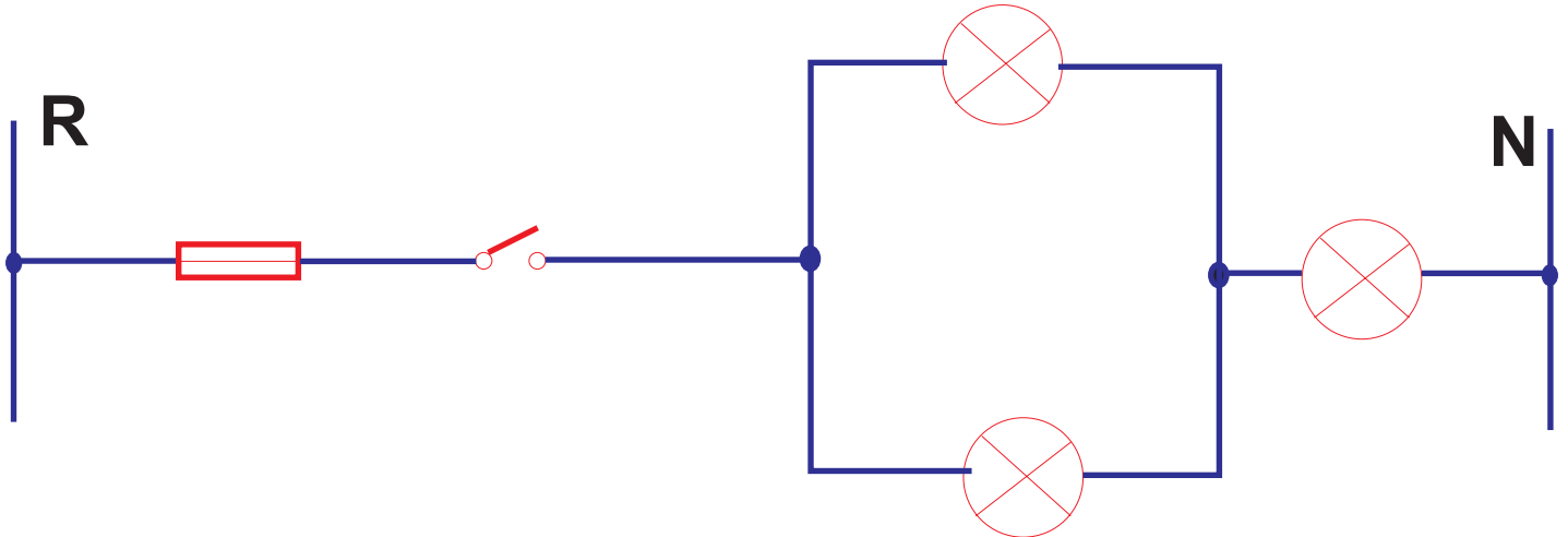
Esquema de conexiones
