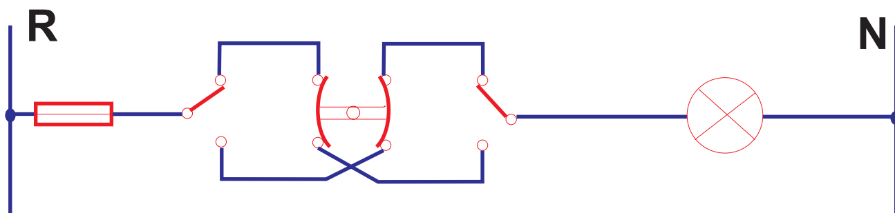
Esquema de conexiones
